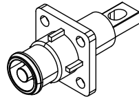
RES-P-10/25-D-B-20-0G(BK) 板接式 (腰形孔) BUSBAR TYPE
