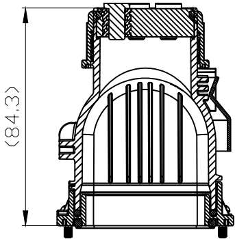
剖视图 A-A
